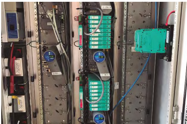
MODERNIZACIÓN DE INFRAESTRUCTURA FIELDBUS
