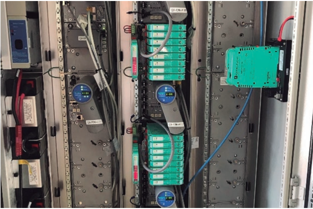
MODERNIZACIÓN DE INFRAESTRUCTURA FIELDBUS
