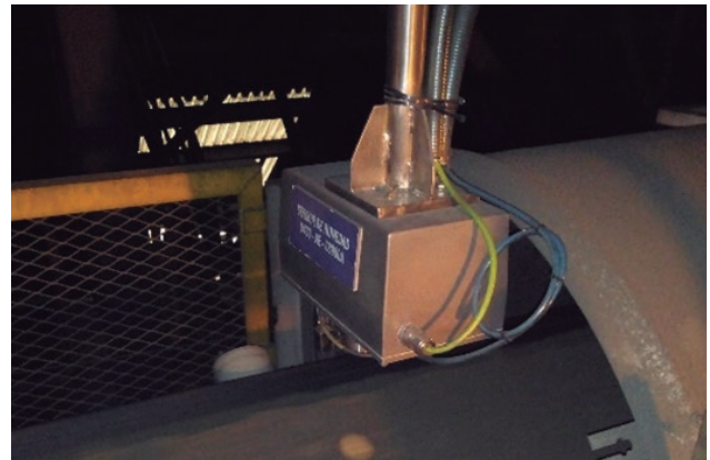
PUESTA EN MARCHA Y CALIBRACIÓN DE ANALIZADOR DE HUMEDAD DE CONCENTRADO DE COBRE
